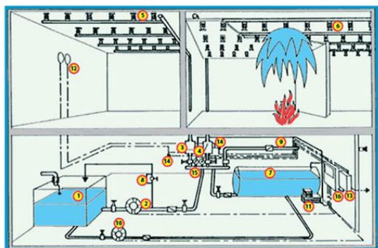
Sistem za automatsko gašenje požara (sprinkler sistem)
